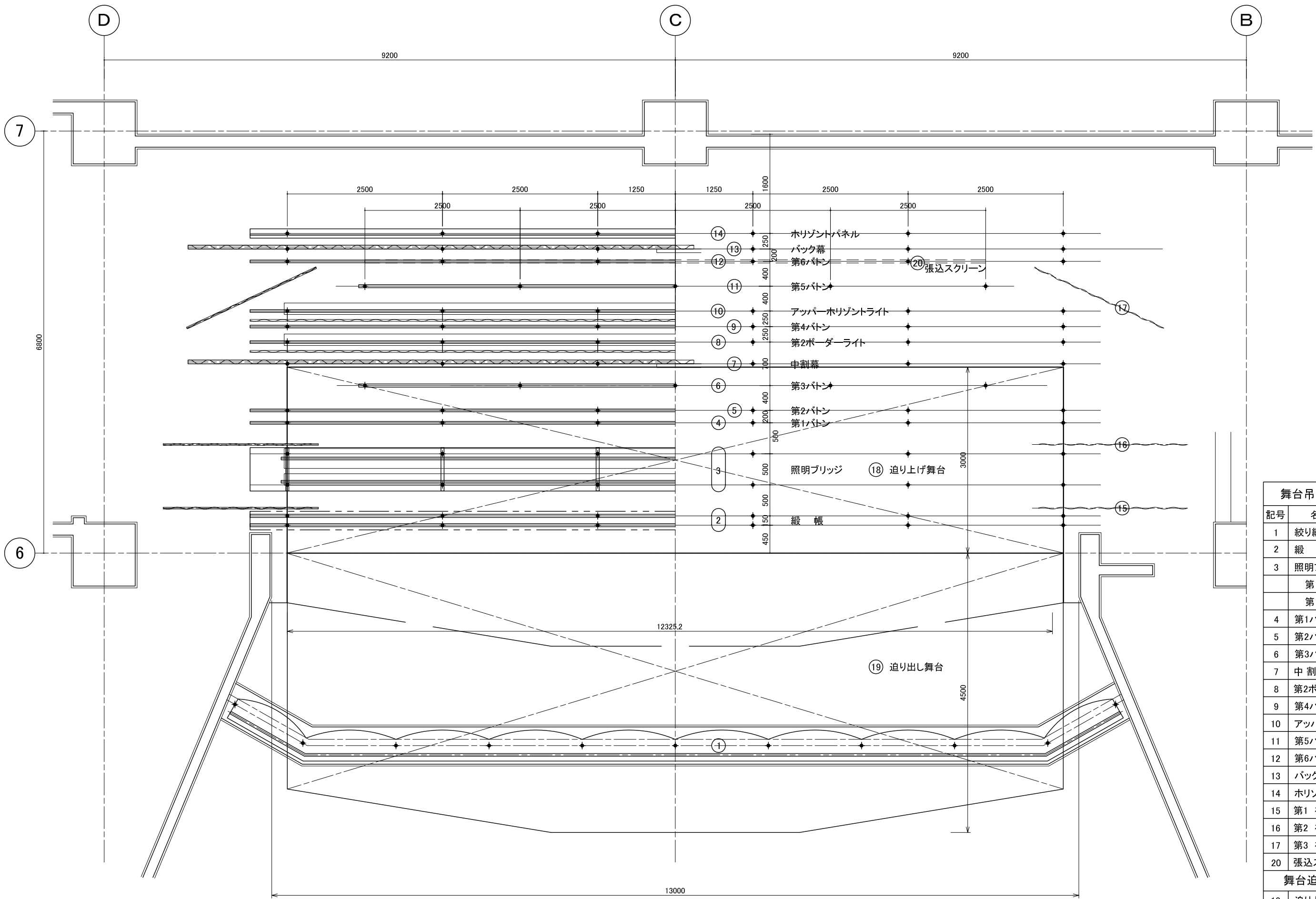
舞台機構設備平面図 S=1/30
